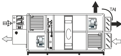
kuvassa vasenkätinen kojemalli (L) pyörivällä lämmönsiirtimellä
